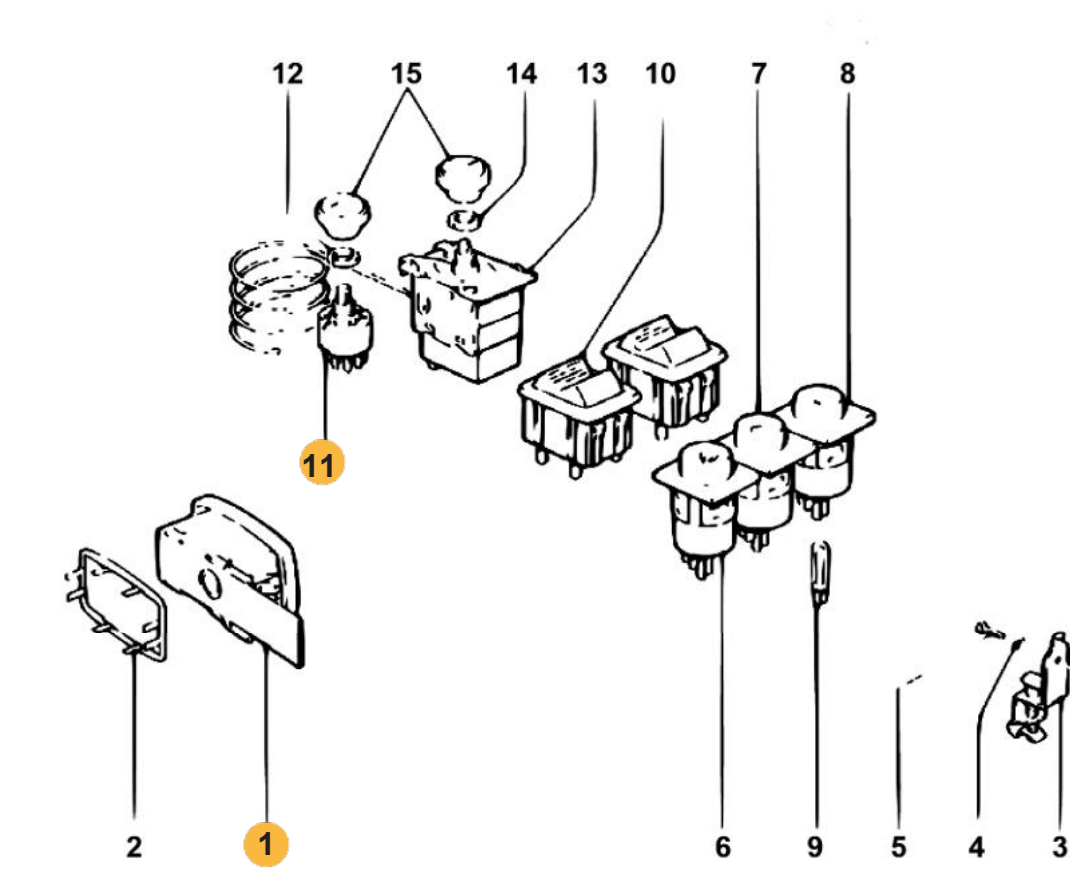
Spiegelschalter
