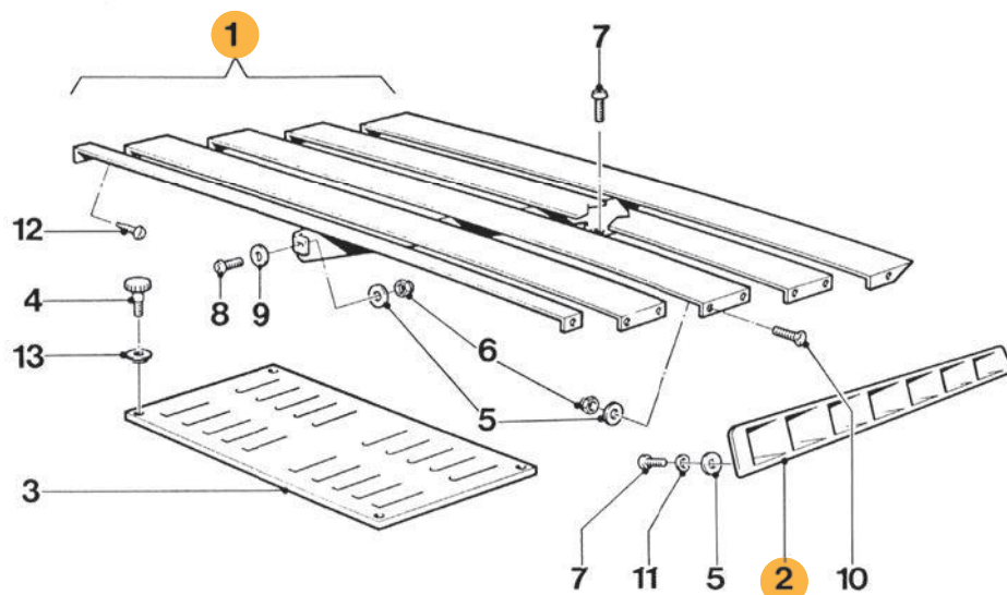
Hecklamellen
