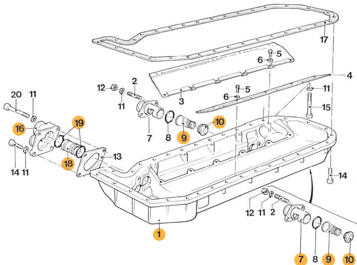
Ölwanne
