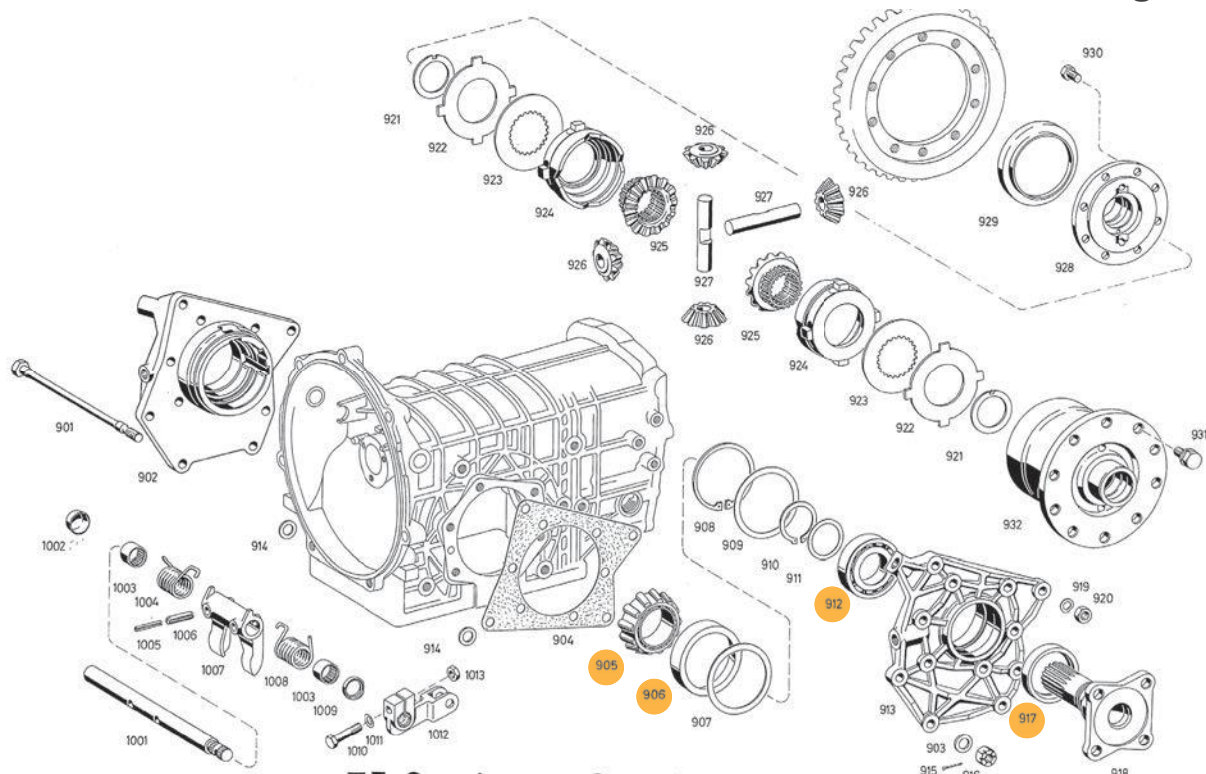
ZF-Synchroma-Getriebe 5 DS 25/2
