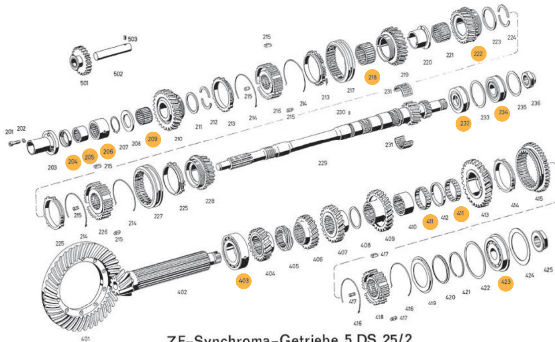
ZF-Synchroma-Getriebe 5 DS 25/2
